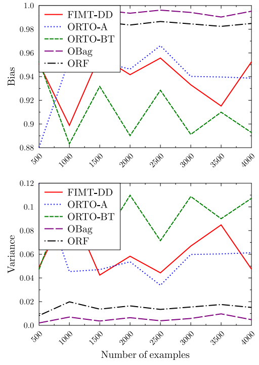
(d) Winequality
